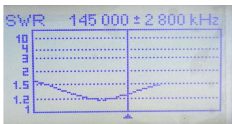
SWR graf za 145.000
