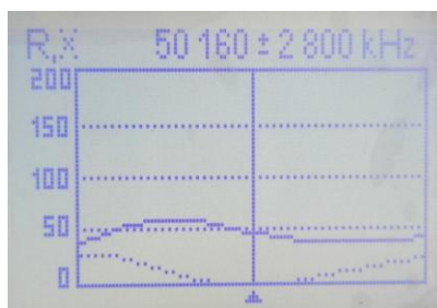
R, X graf
